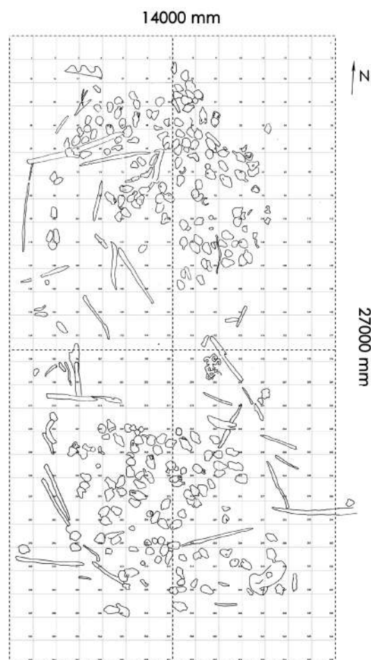
Рис. 3. Графический план кораблекрушения XI в. у Балаклавы.
