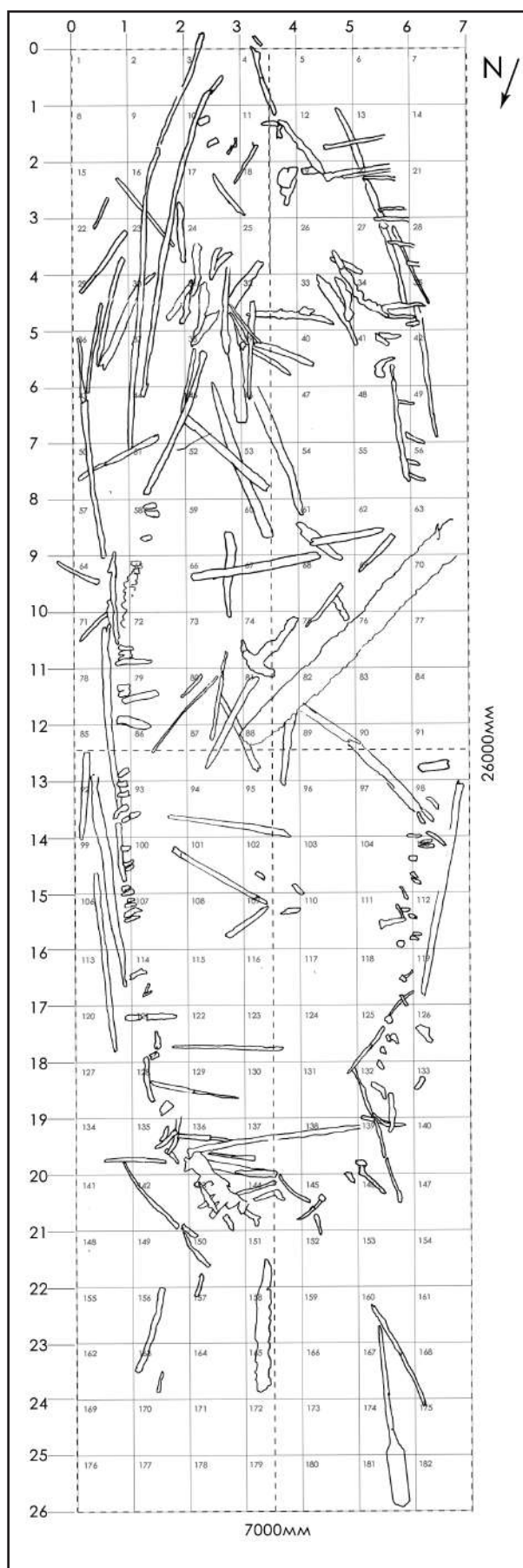
Рис. 6. Графический план кораблекрушения XI–XII вв. у Балаклавы.
