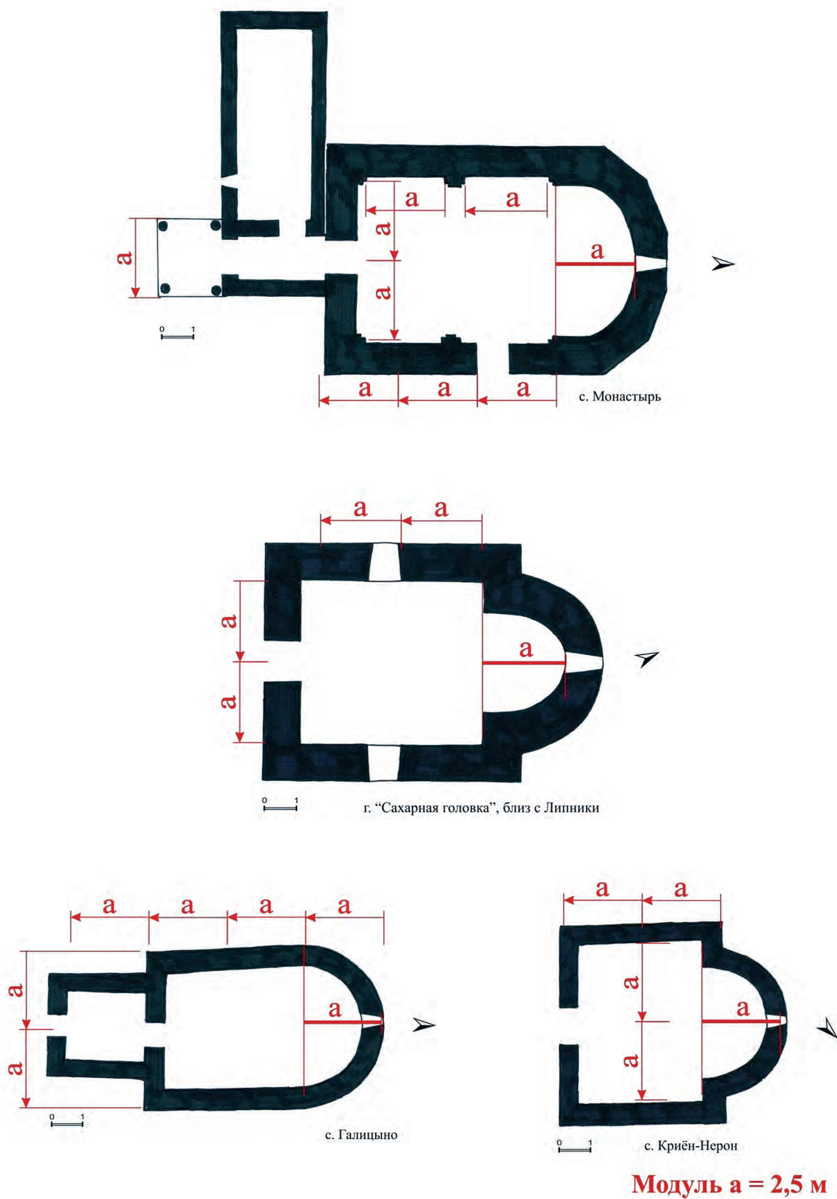
Рис. 1. Модульный размер в храмах Причерноморской Зихии, VIII–IX вв.
