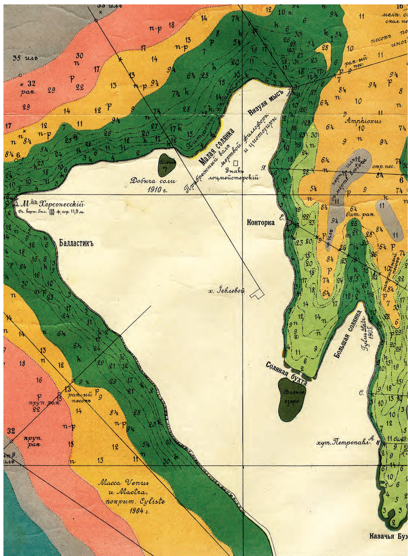
Рис.1. Район Маячного полуострова и Казачьей бухты на карте С.А.Зернова 1912 г.
