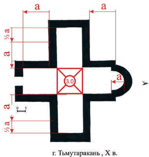
Рис. 2. Совпадение модульных размеров храмов типа «свободный крест» в Алании (X в.), Тьмутаракани (X в.) и в раннехристианских храмах-усыпальницах Херсонеса
