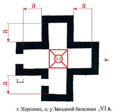
Рис. 2. Совпадение модульных размеров храмов типа «свободный крест» в Алании (X в.), Тьмутаракани (X в.) и в раннехристианских храмах-усыпальницах Херсонеса
