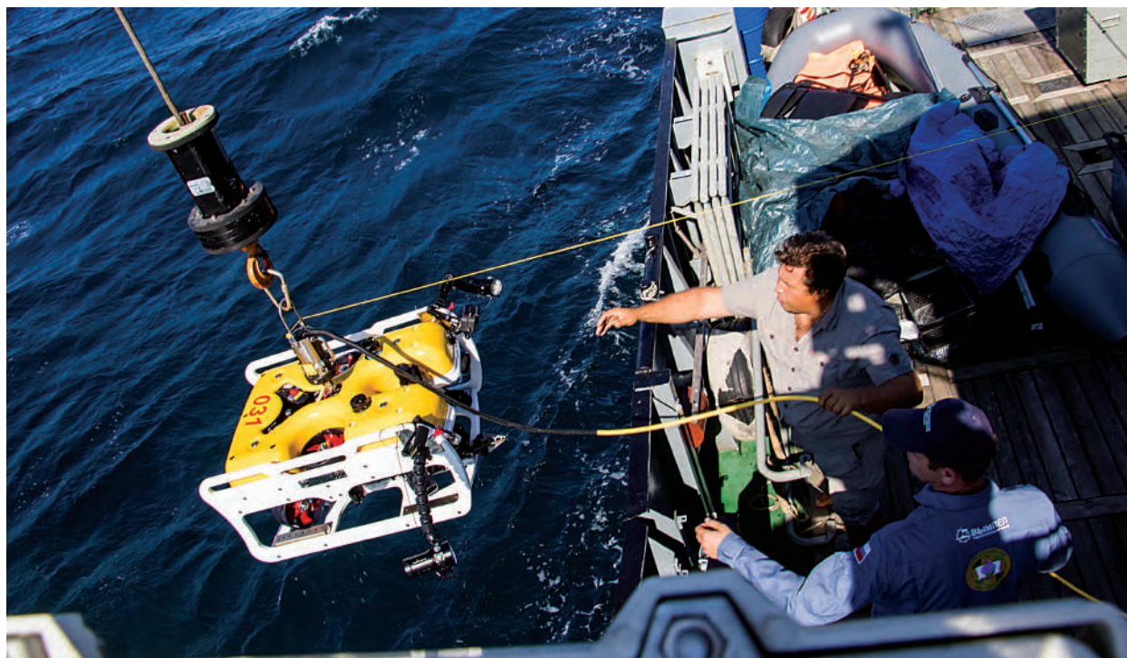
Рис. 1. ТНПА с дополнительным навесным оборудованием при спуске в воду.
